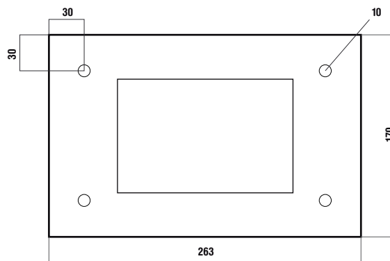
Base Vint 600
