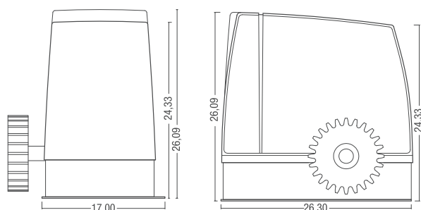
Medidas Vint 600
