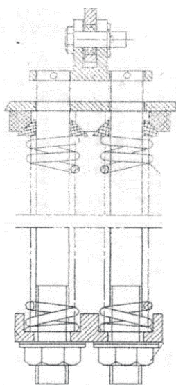
Resorte para contrapeso
