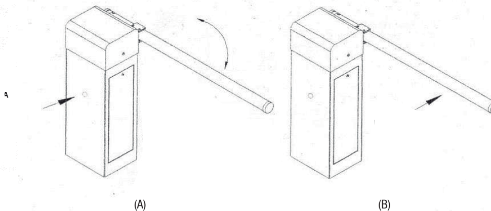
Inserte la llave de desbloqueo, gírela en sentido antihorario para liberar el embrague y operar la barrera manualmente
